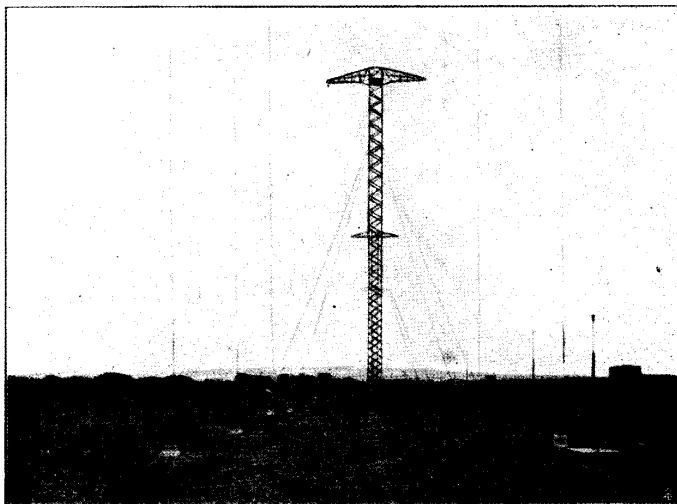
STAZIONE TRASMITTENTE A FASCIO DI BRIDGWATER COSTRUITA DALLA MARCONI'S WIRELESS TELEGRAPH COMPANY LTD. PER L'UFFICIO GENERALE POSTE INGLESÌ SU SISTEMA MARCONI ONDE CORTE.
